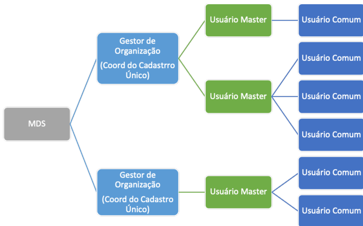
Figura 1 - Fluxo do Gerenciamento de Identidade e Acesso
